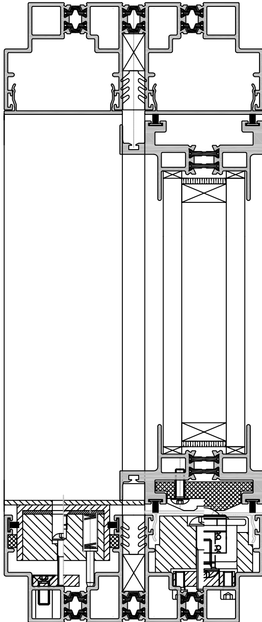
VERROUILLAGE PAR CAPOT MOBILE
