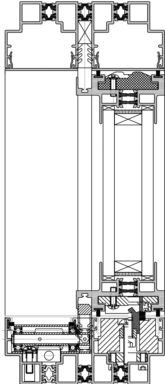
VERROUILLAGE PAR CREMAILLIERE
