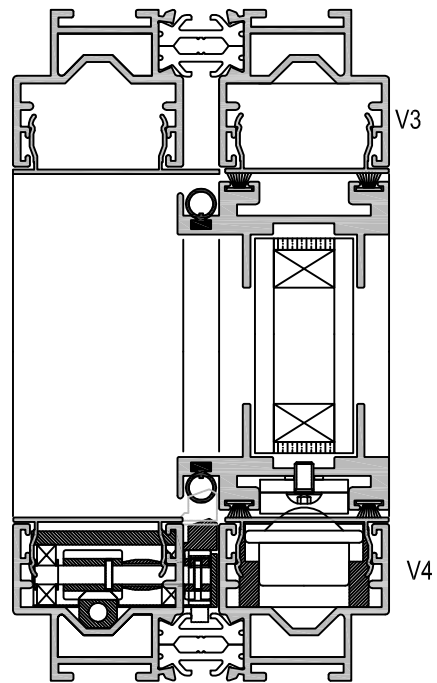
VERROUILLAGE PAR CREMAILLERE
