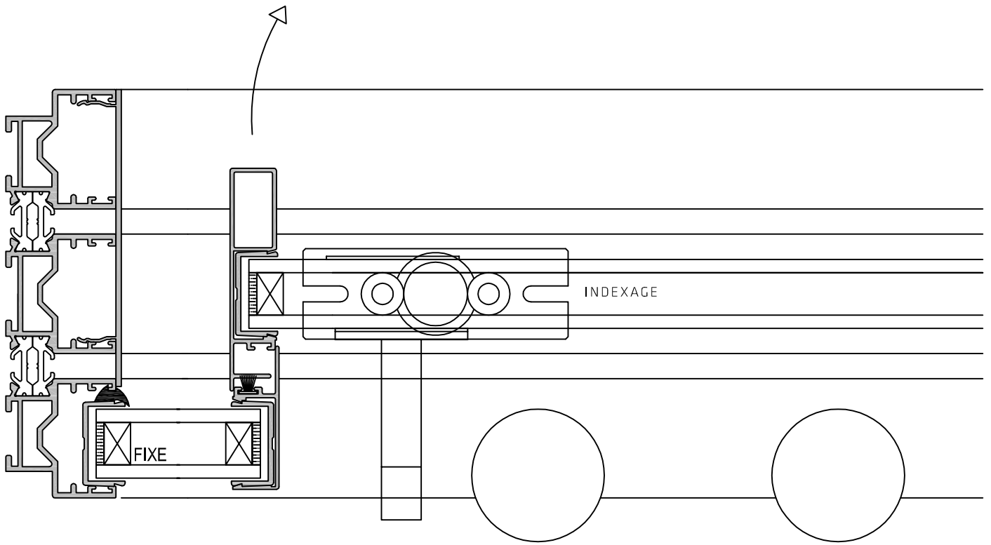
BOUTONS DE VERROUILLAGE ET D'ETANCHEITE AU PIED
