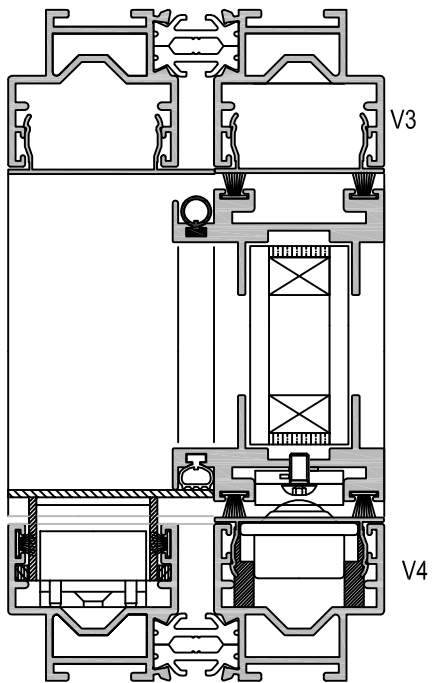
VERROUILLAGE PAR CAPOT MOBILE
